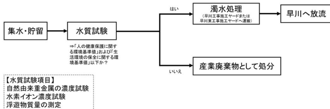
図 5-1 排水処理のフロー
