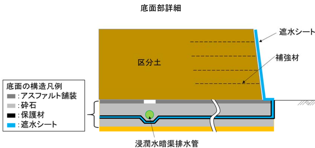
図 2-3(2) 湯島地区（田島）発生土仮置き場における盛土計画
