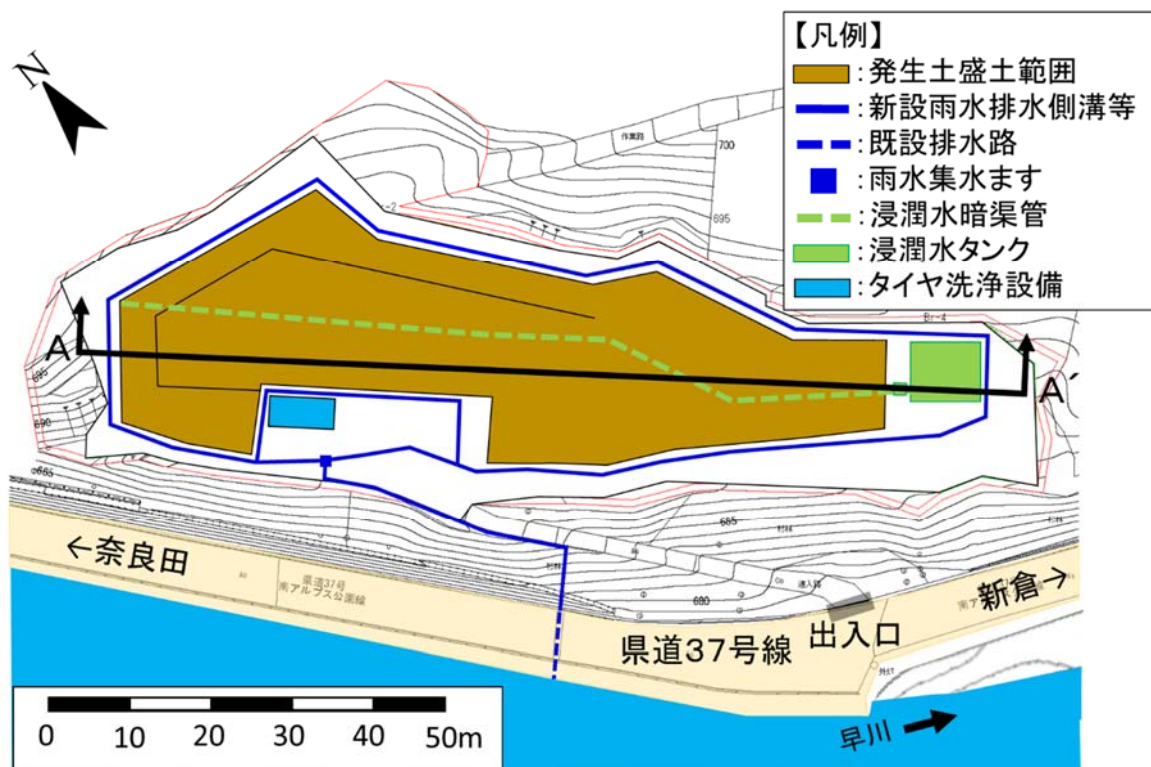
平面図
