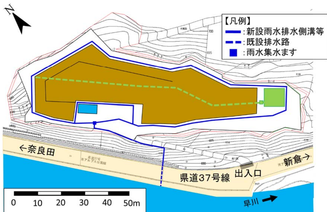
図 5-2 湯島地区（田島）発生土仮置き場の雨水側溝
