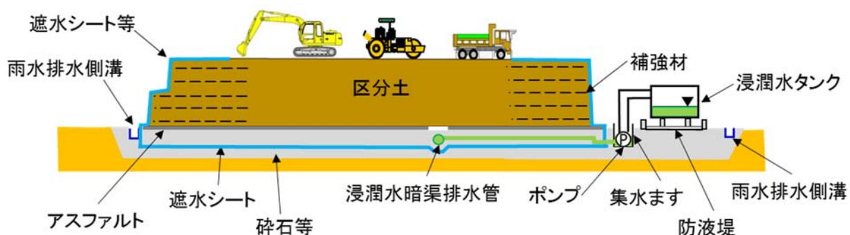
図 5-3 湯島地区（田島）発生土仮置き場における計画（区分土搬入中）
