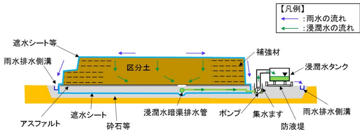
図 5-4 湯島地区（田島）発生土仮置き場における計画（仮置き期間中）
