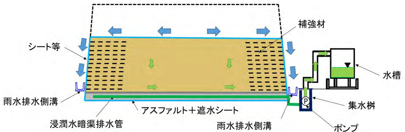
図 5-3 湯島地区発生土仮置き場における計画のイメージ（区分土搬入中）
