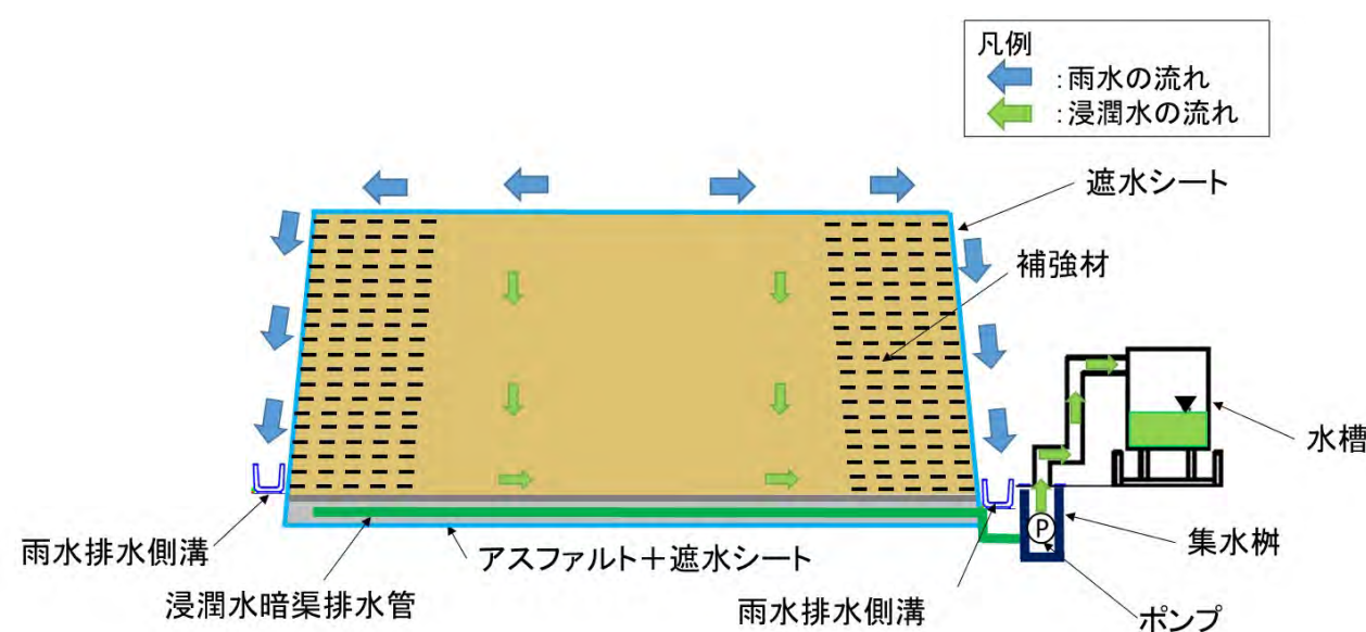
図 2-4 排水計画概要図
