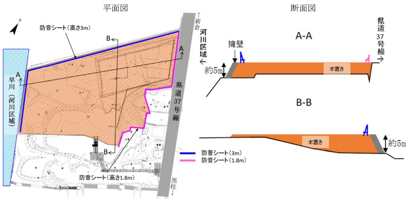
図 2-3 発生土置き場における盛土計画（本置き時（施工中））
