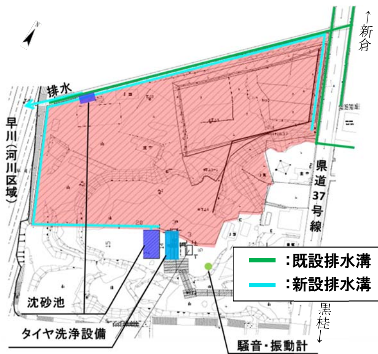
図 3-4 水環境に関する計画面の環境保全措置（工事中）
