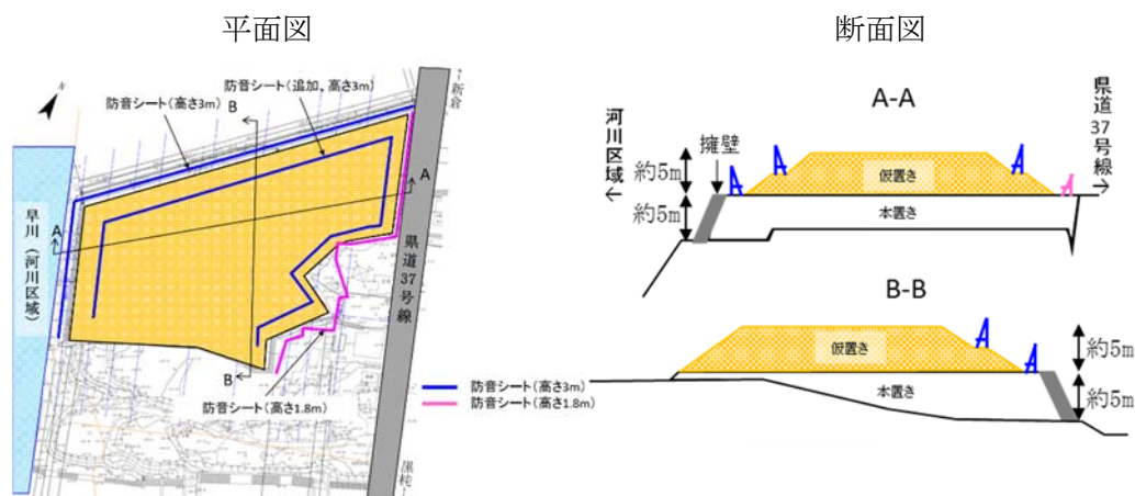
図 3-7 大気環境に関する計画面の追加の環境保全措置（仮置き時）
