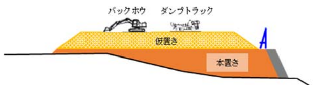
図2-5 発生土置き場における主な施工手順
