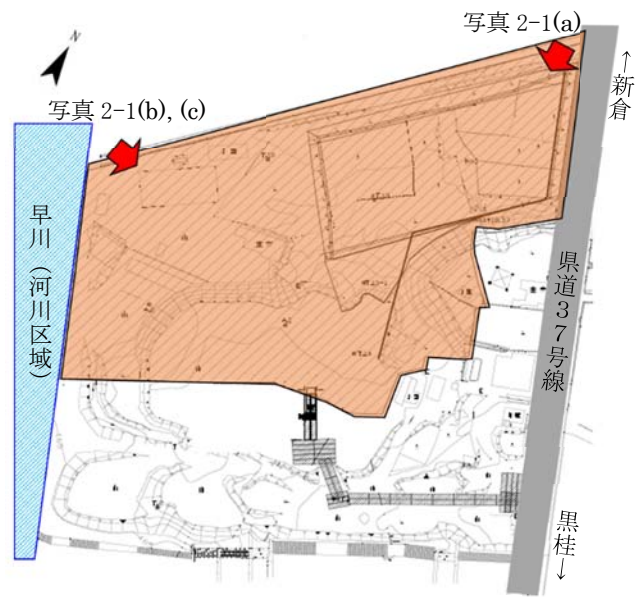
図 2-2 塩島地区発生土置き場平面図
