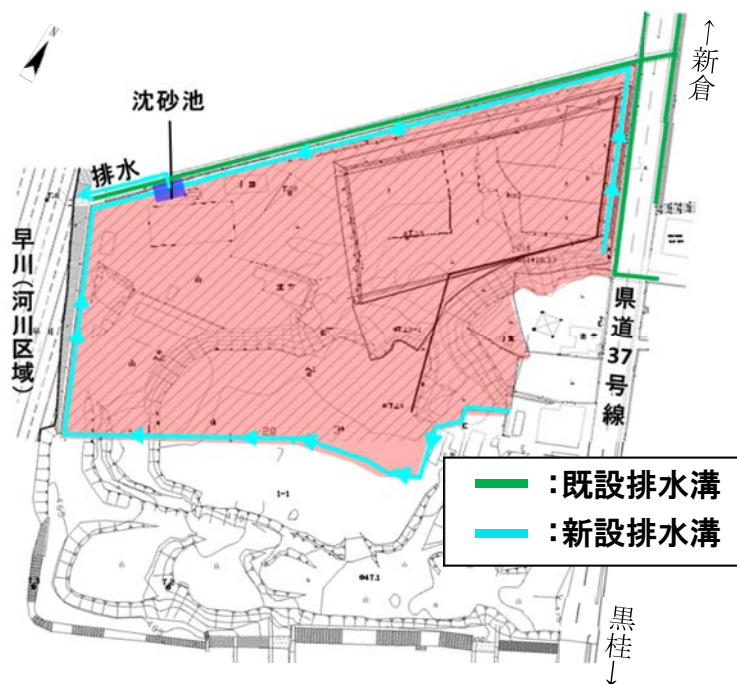
図 3-5 水環境に関する計画面の環境保全措置（仮置き土搬出後）
