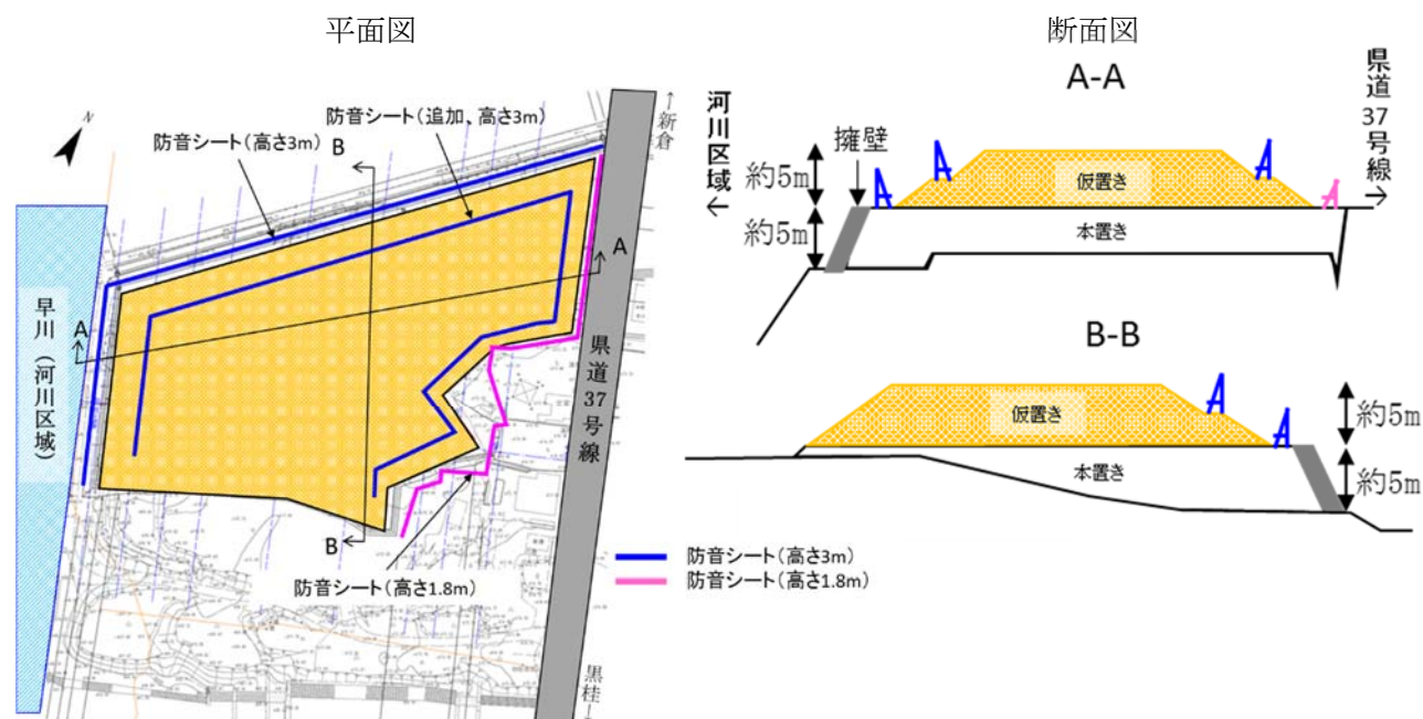
図 2-4 発生土置き場における盛土計画（仮置き時）
