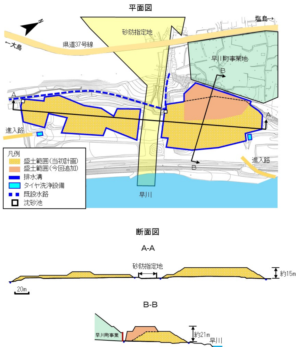
図2-3 西之宮地区発生土仮置き場における盛土計画
