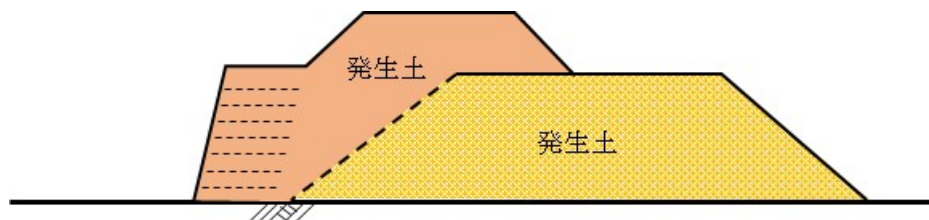
図 2-4(2) 西之宮地区発生土仮置き場における主な施工手順（仮置き）
