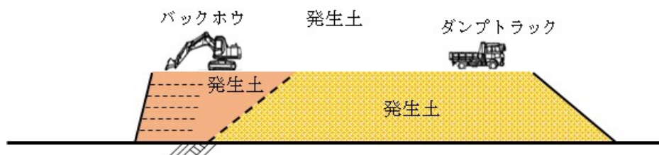
図 2-4(3) 西之宮地区発生土仮置き場における主な施工手順（発生土搬出）
