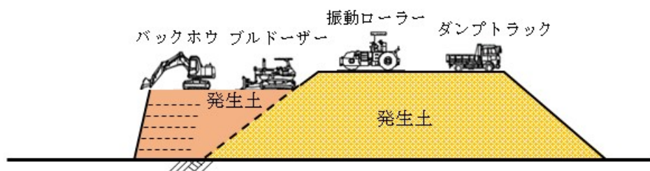
図 2-4(1) 西之宮地区発生土仮置き場における主な施工手順（発生土搬入、締固め）
